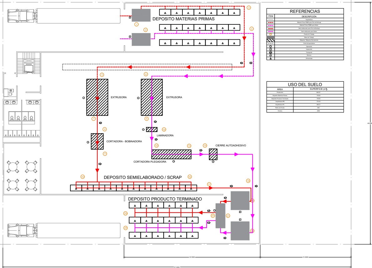
PLANTA BAJA
