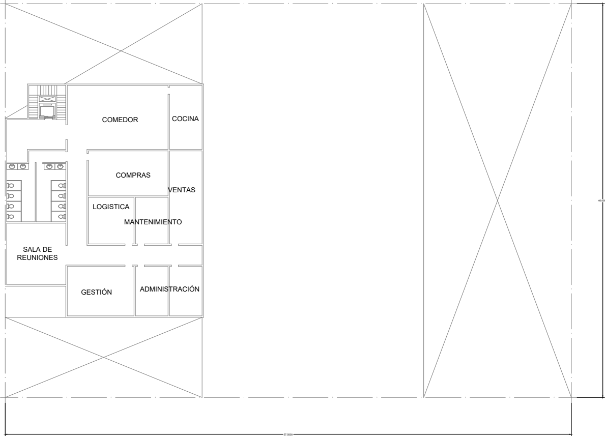
PLANTA ALTA
